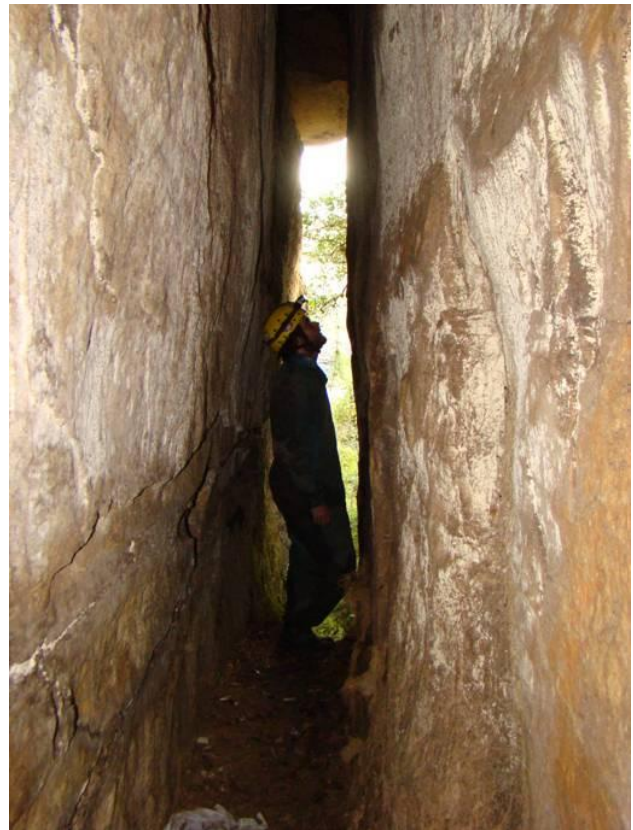
Figura 14: típica galeria estrutural – Caverna da Chaminé – Canyon do Rio São Jorge.
